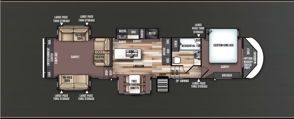
372RD FLOORPLAN
