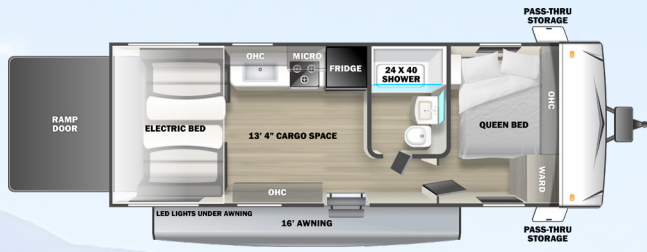
21RQMX (13' 4" CARGO)
