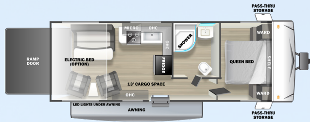
24FS (13' CARGO)
