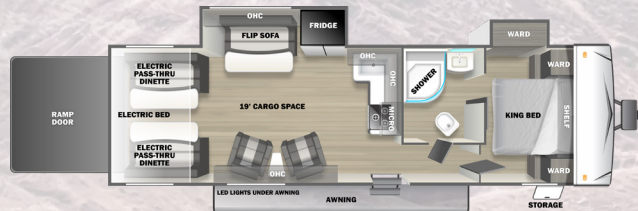
30FKGDX (19' CARGO)
