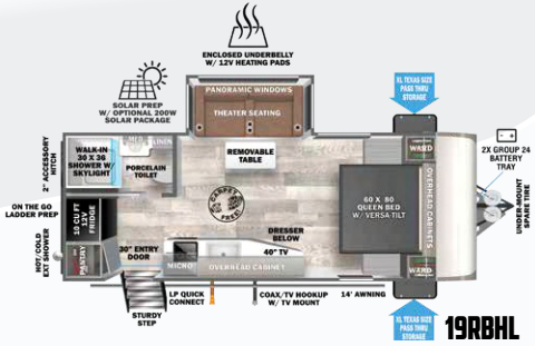
19RBHL UVW = 5 403 lb Longueur = 24 pi
