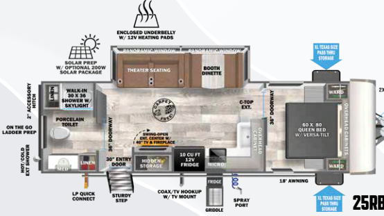
25RBHL UVW = 6 678 lb Longueur = 30 pi 10 po
