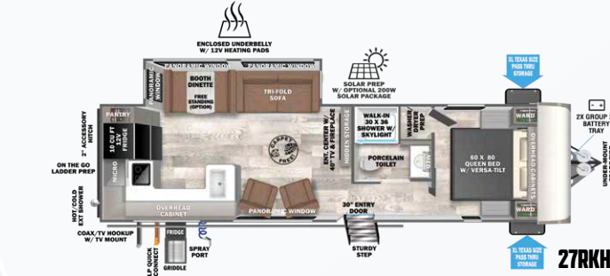
27RKHL UVW = 6 758 lb Longueur = 34 pi
